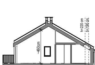
Schematyczny przekrój
